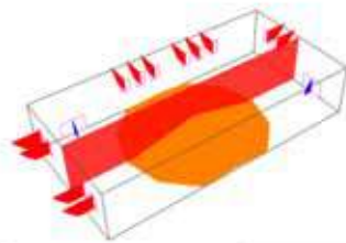
MODELLO CFAST - TEMPERATURA DELLA ZONA SUPERIORE PARETI E SOLAIO IN LATERIZIO
