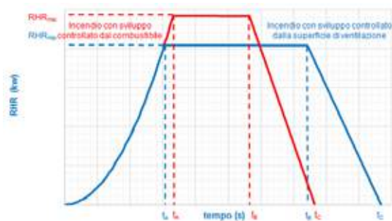
DIFFERENZE TRA INCENDI CONTROLLATI DAL COMBUSTIBILE E DALLA SUPERFICIE DI VENTILAZIONE
